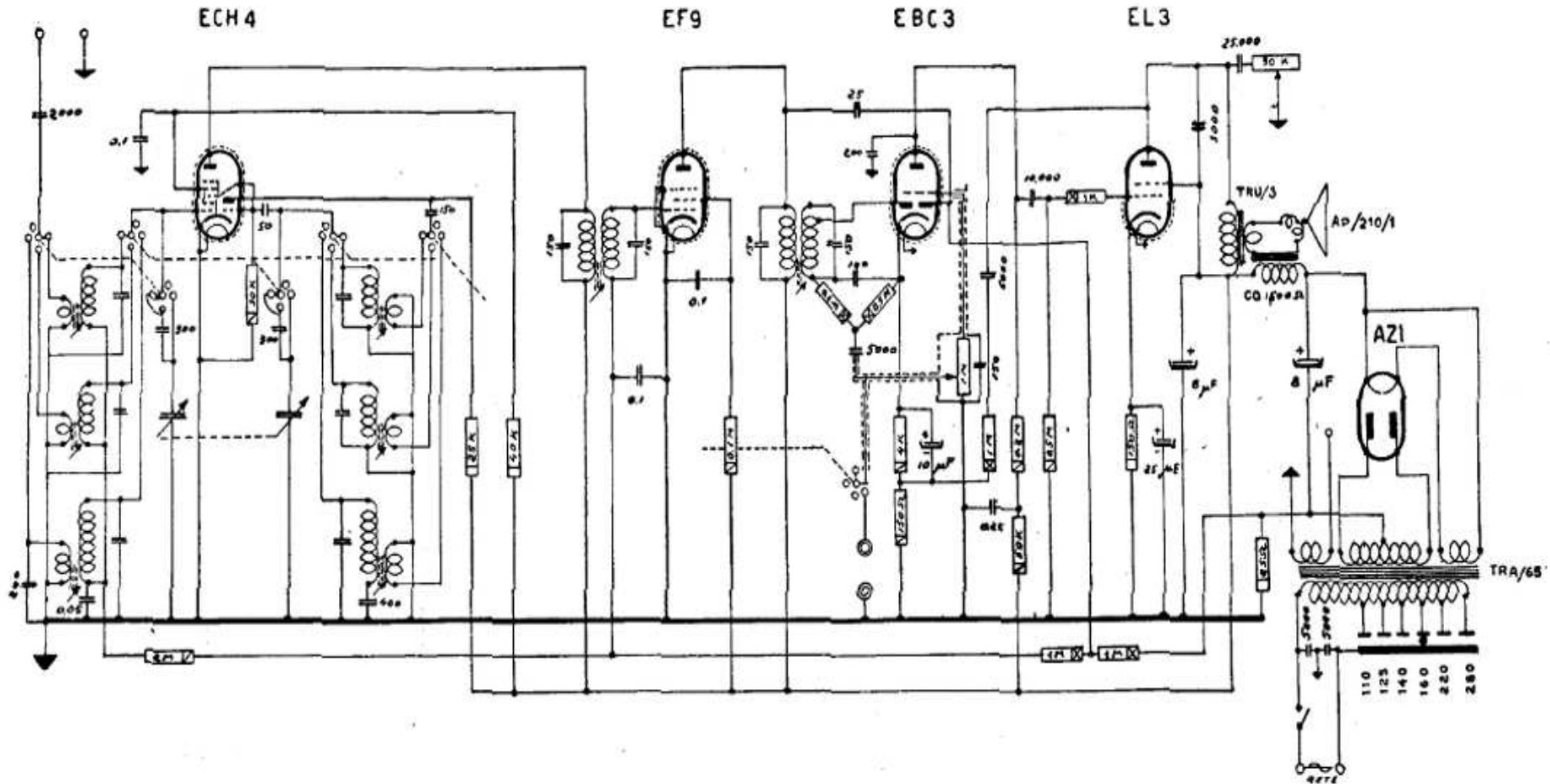
BERTONCINI RADIO - Mod. LEILA 1 - Una gamma onde medie, due gamme onde corte, Reazione negativa al catodo della EBC3. Media frequenza: 468 kc. Sensibilità media: 20 \mu V. Bobina campo: 1500 ohm. Potenza d'uscita: 3 watt.
